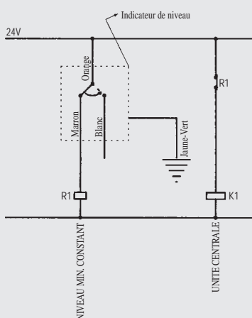
1.1 Niveau minimum constant
