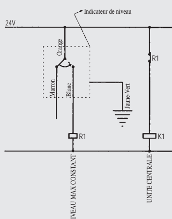
1.2 Niveau maximum constant
