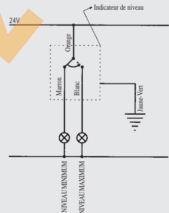
1.3 Signal niveau minimum et maximum
