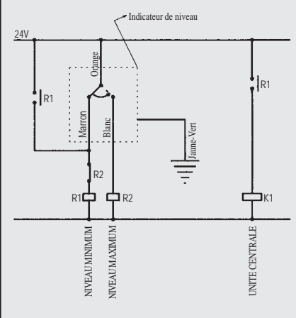
1.3 Niveau entre maximum et minimum
