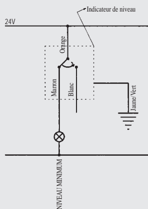
1.1 Signal niveau minimum
