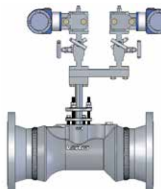
Transmetteur double
