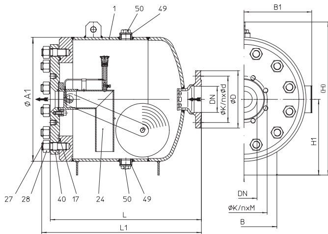
Fig. 637....1 à brides -
