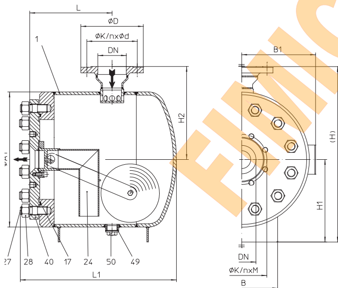
Fig. 638....1 Exécution équerre à brides -
