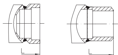
Fig. 631....3 à manchons à souder
