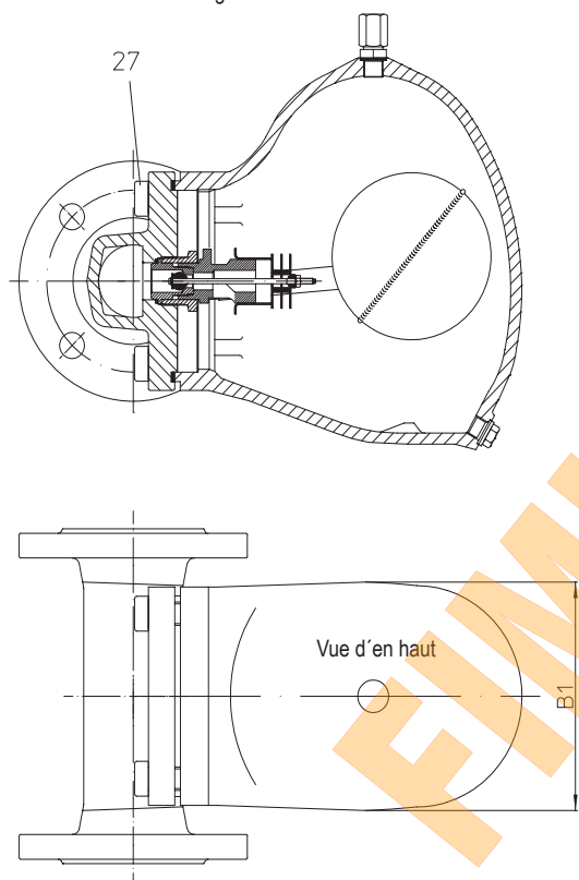
Fig. 630....1 à brides - montage vertical
