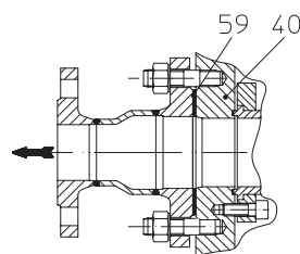
Exécution côté sortie pour DN50
