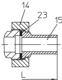
Fig. 610....5 à raccord union à souder
