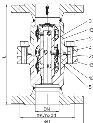
Fig. 616....1....10K2 (DN40-50) avec 10 capsules - Type in-line, à brides
