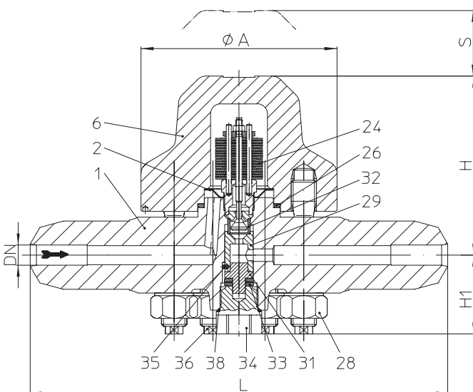
Fig. 600....4 à embouts à souder
