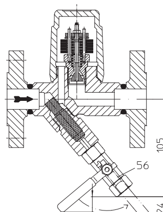
Robinet à tournant sphérique comme robinet de purge avec filtre intégré (limité jusqu'à 232psi, 410°F / 16bar, 210°C)
