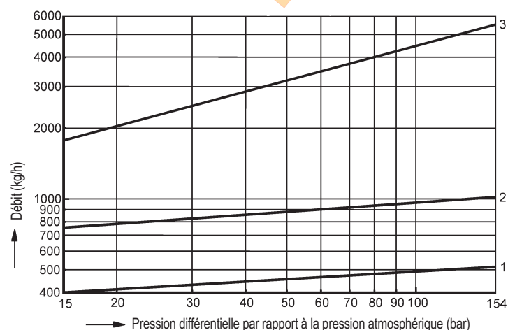
Diagramme de débit PN250
