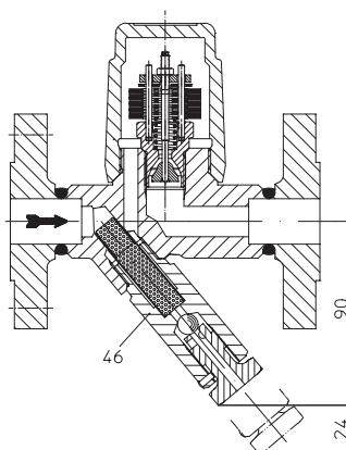
Robinet de purge avec filtre intégré
