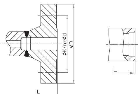
Fig. 600....1 (PN400) à brides
