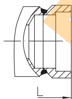
Fig. 600/601....3 à manchons à souder
