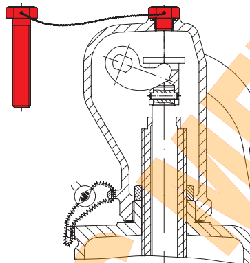
Vis de blocage
