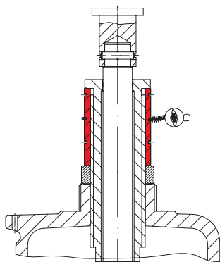
Manchon d'arrêt
