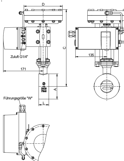
avec positionneur électro-pneumatique
